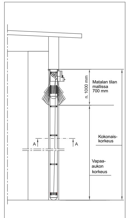
Asennusmitat
